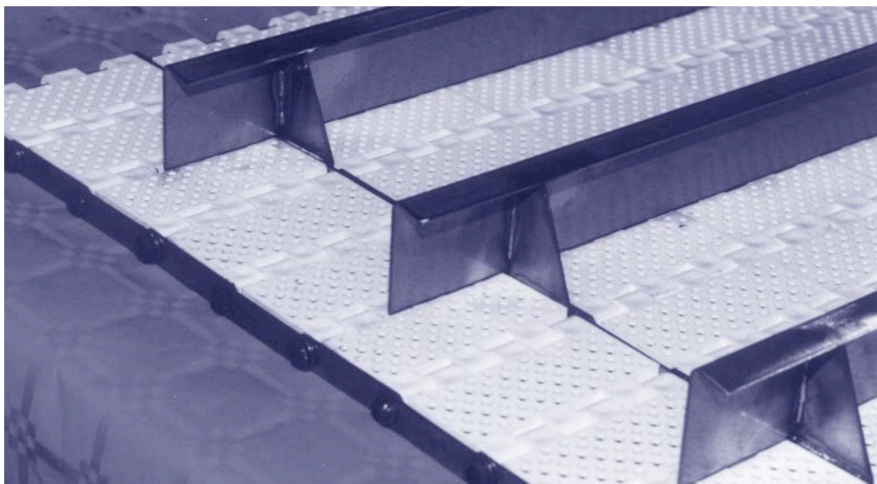
MT-E-KK kunststof modulen band met RVS meenemers
