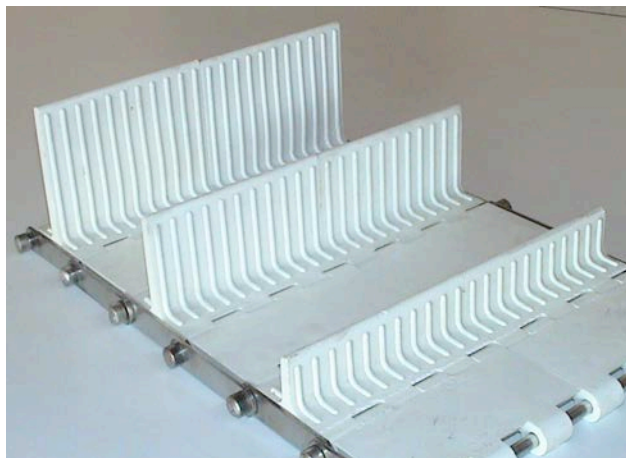
MT-E modulen band met geïntegreerde plastic meenemers
