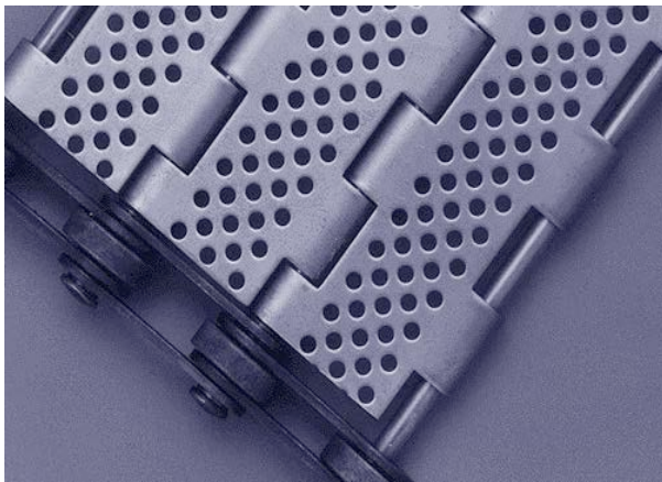
Voorbeeld van een SC-HK scharnierplatenband met zijketting en perforatie
