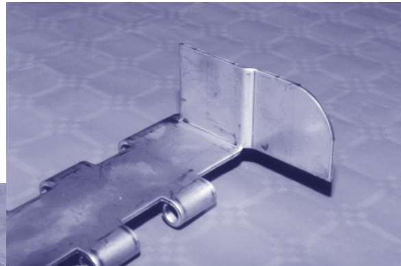
steek 63 mm
